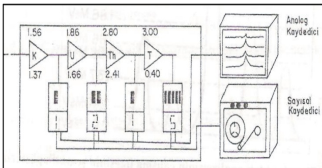
Şekil 5.10. Kanal Sayısı 4 Olan Bir Spektromet Ve Kaydedicinin Şematik Gösterimi.
