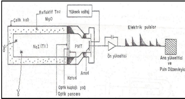
Şekil 5.8. Gamma Işınları Algılayıcısının Şematik Gösterimi (Aydın 2004).
