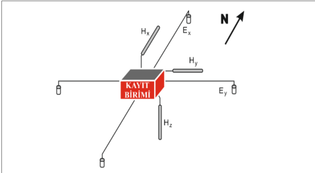
Şekil 6.4. Elektrik (E) Alanın İki Ve Manyetik (H) Alanın Üç Bileşeninin Coğrafi Yönere Göre Ölçümü. (x kuzey-güney, y doğu-batı ve z düşey yönü göstermektedir.)
